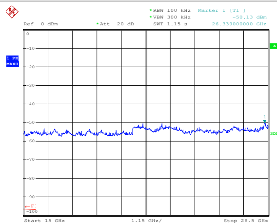
Plot 6 (15÷26.5GHz)
