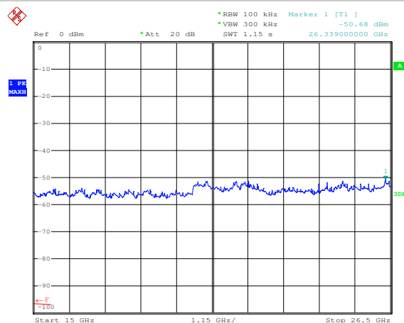
Plot 6 (15÷26.5GHz)
