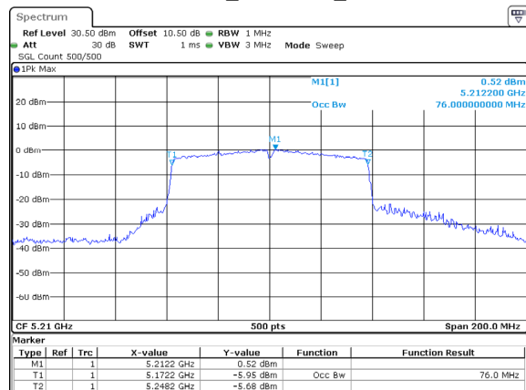
802.11ac80_5210MHz_Chain 2
