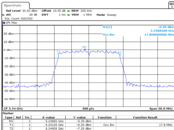
802.11ac20_5240MHz_Chain 1
