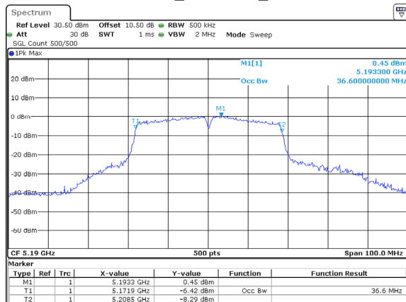
802.11ac40_5190MHz_Chain 2
