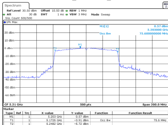
802.11ac80_5210MHz_Chain 1
