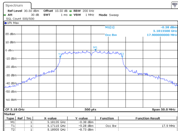
802.11ac20_5180MHz_Chain 2
