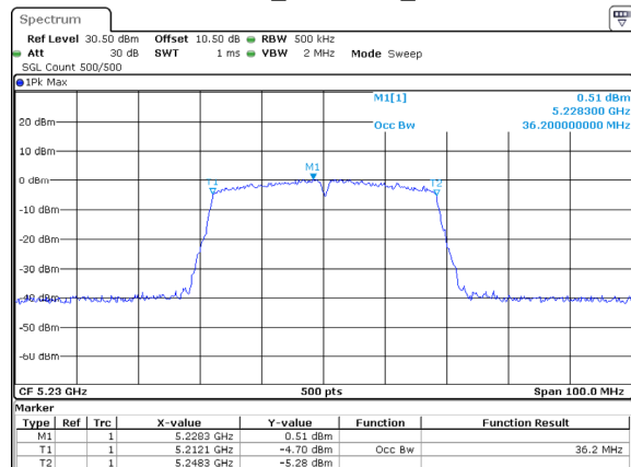
802.11ac40_5230MHz_Chain 2
