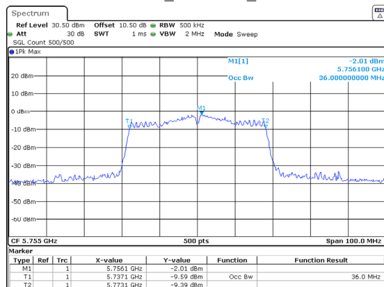
802.11ac40_5755MHz_Chain 1
