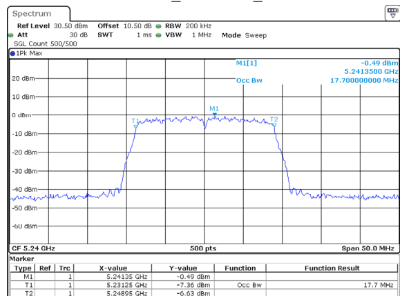
802.11ac20_5240MHz_Chain 2
