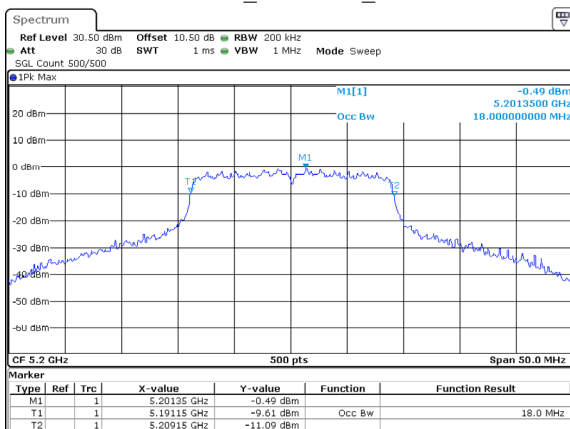
802.11ac20_5200MHz_Chain 2
