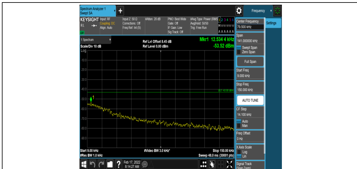
Band26-3MHz-QPSK-26740-1-0-Low-0.009-0.15--53.52-PASS
