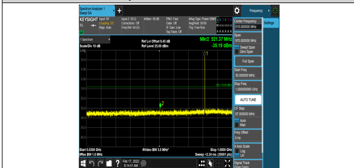
Band26-3MHz-QPSK-26740-1-0-Low-30-1000--35.19-PASS
