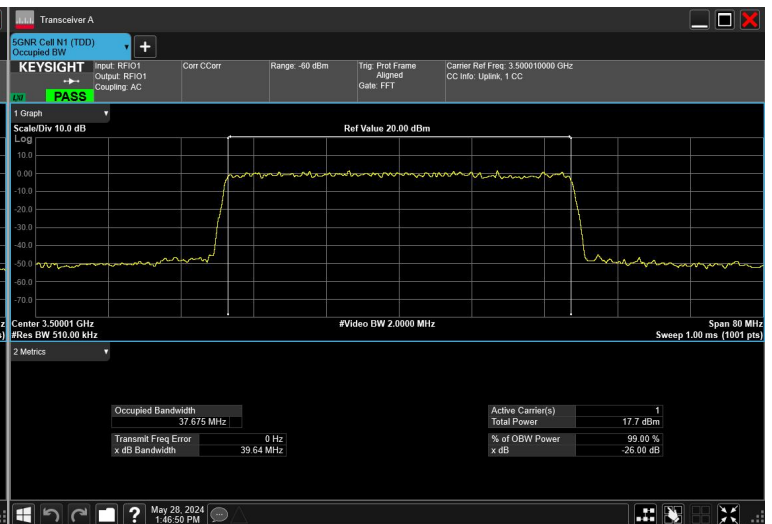
40MHz_30kHz_3500MHz_CP-OFDM QPSK_RB106@0
