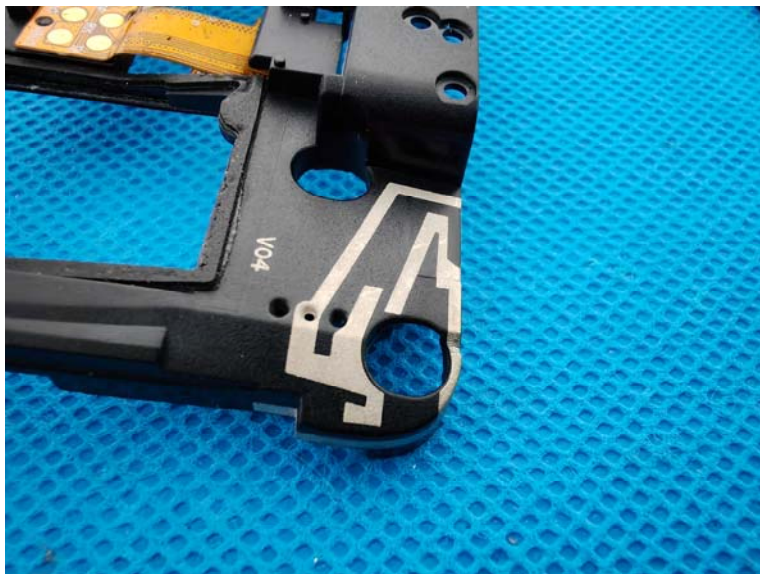
3IN1 ANT
