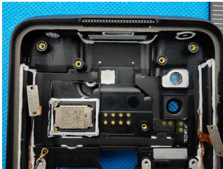
NFC ANT
