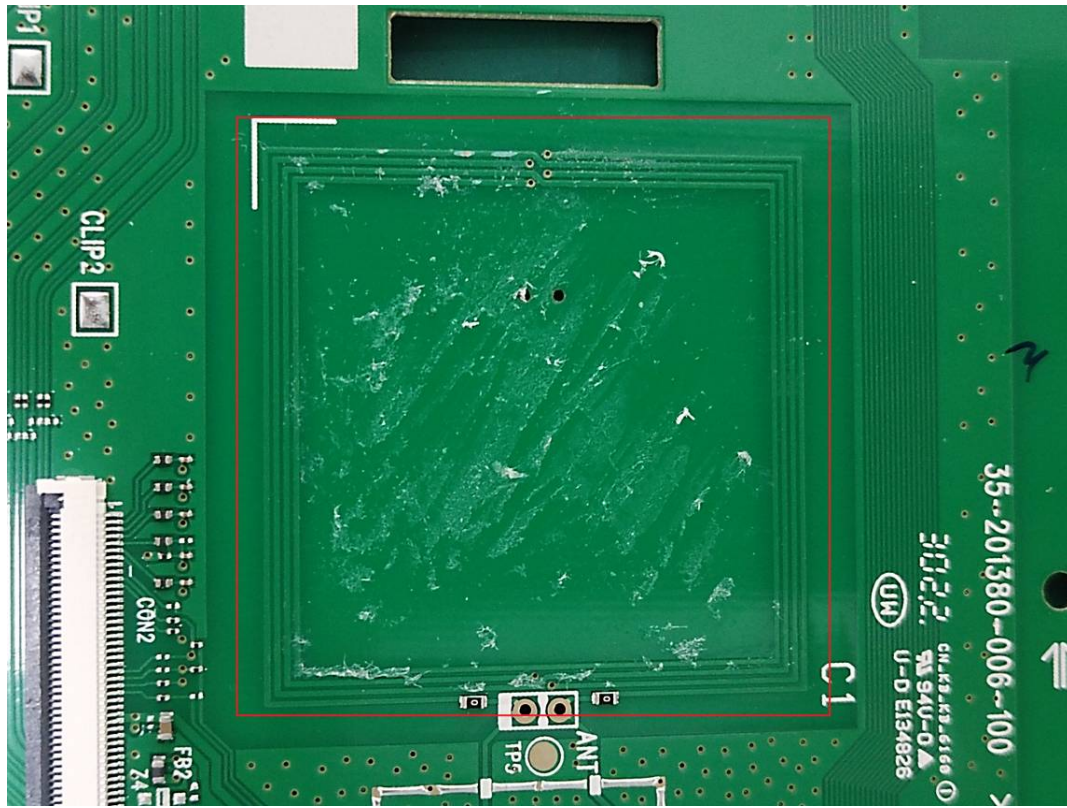
NFC ANT
