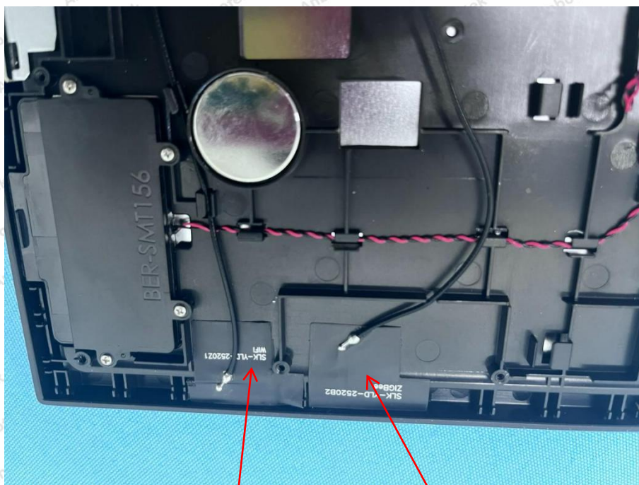
BT&WIFI ANT
