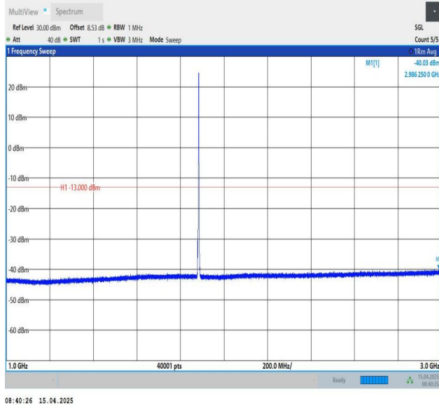
Band25-3MHz-QPSK-26365-1RB#14-1000~3000-PASS
