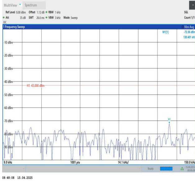
Band25-10MHz-QPSK-26365-1RB#0-0.009~0.15-PASS
