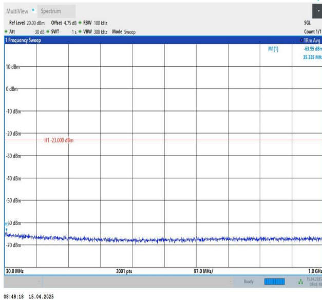
Band25-10MHz-QPSK-26365-1RB#0-30~1000-PASS
