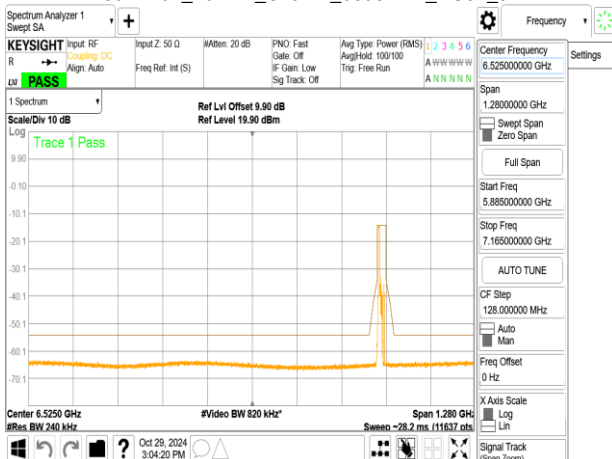
802.11ax_20MHz_ChainB_6895MHz_RU52_37
