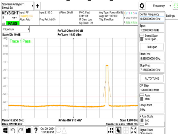
802.11ax_20MHz_ChainB_6855MHz_RU106_54
