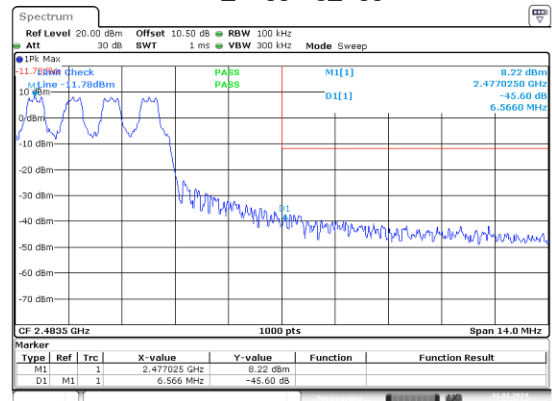
GFSK_Hopping_Upper
