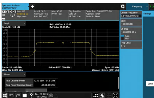
11AC80SISO-Ant0-5610-TPC_L-PASS
