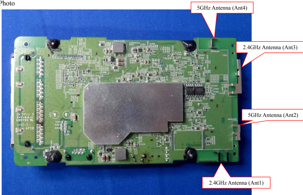
(20) EUT Photo
