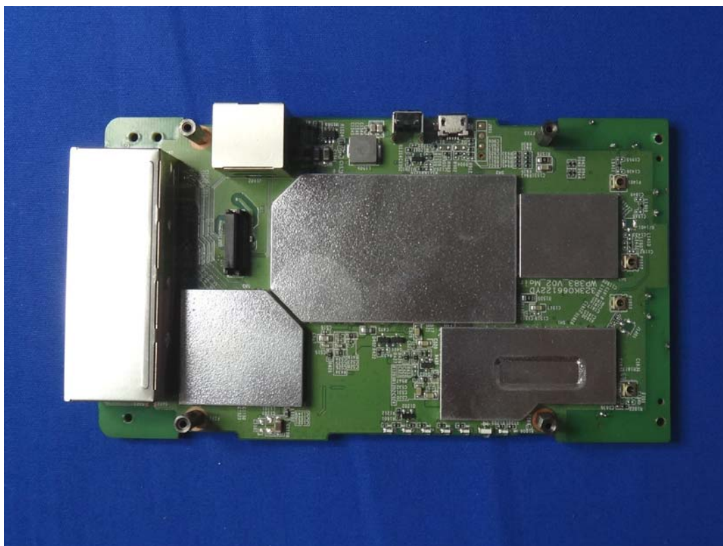
(13) EUT Photo
