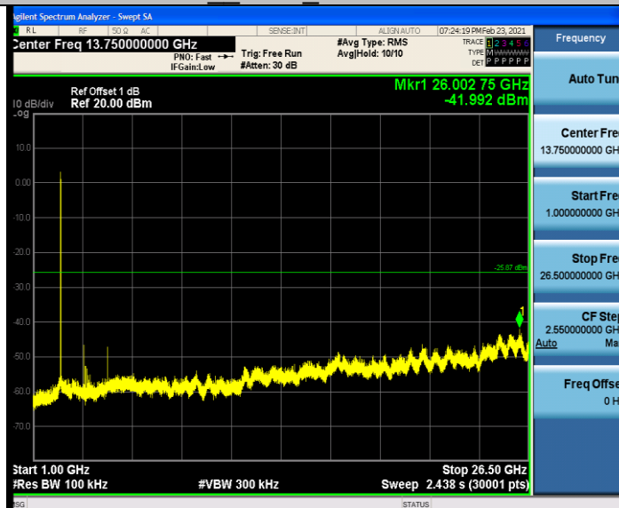
11B 2412 1000~26500
