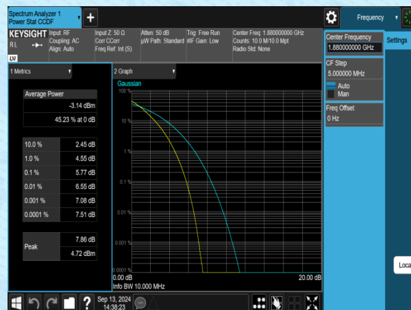
Band2-10MHz-QPSK-18900-50RB#0-PASS
