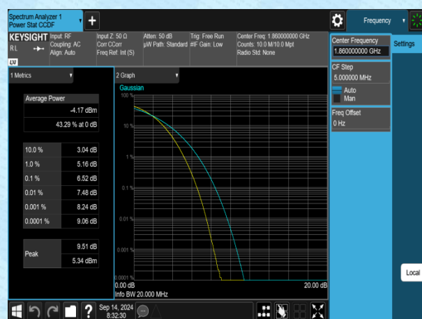
Band2-20MHz-16QAM-18700-100RB#0-PASS
