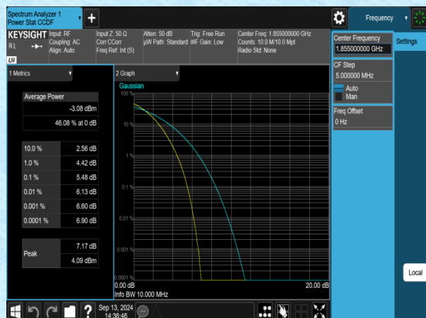
Band2-10MHz-QPSK-18650-1RB#0-PASS
