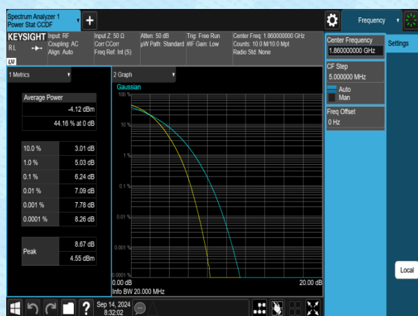
Band2-20MHz-16QAM-18700-1RB#0-PASS
