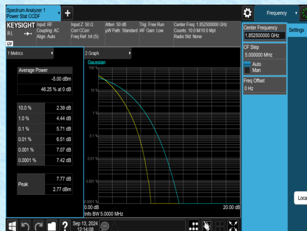
Band2-5MHz-QPSK-18625-25RB#0-PASS
