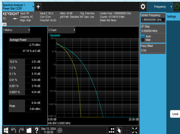
Band2-3MHz-QPSK-18900-1RB#0-PASS
