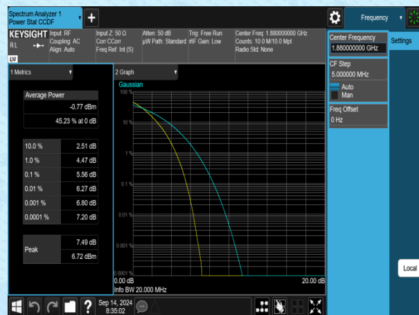
Band2-20MHz-QPSK-18900-100RB#0-PASS
