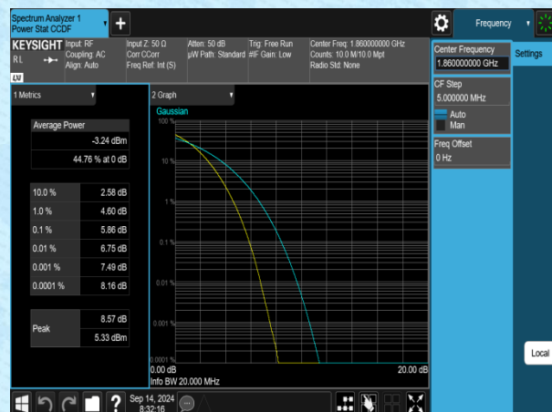
Band2-20MHz-QPSK-18700-100RB#0-PASS
