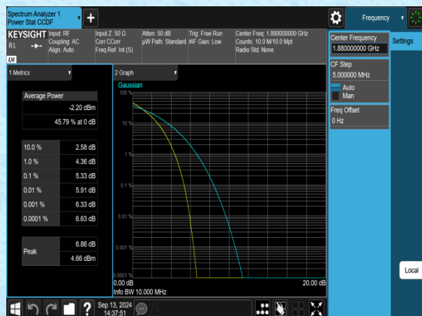
Band2-10MHz-QPSK-18900-1RB#0-PASS
