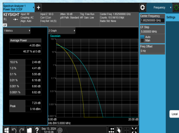
Band2-5MHz-QPSK-18625-1RB#0-PASS
