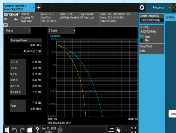
Band2-5MHz-QPSK-18900-25RB#0-PASS
