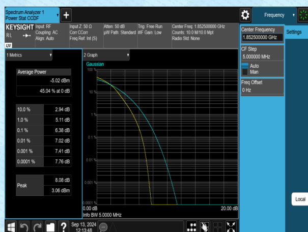
Band2-5MHz-16QAM-18625-1RB#0-PASS
