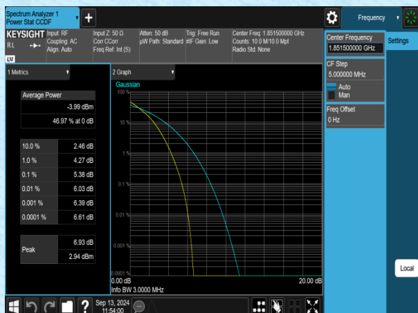
Band2-3MHz-QPSK-18615-1RB#0-PASS
