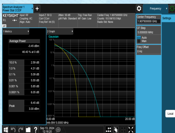
Band2-5MHz-QPSK-19175-1RB#0-PASS
