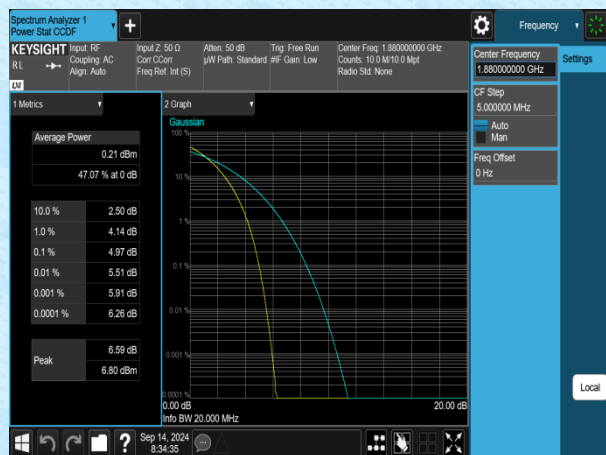
Band2-20MHz-QPSK-18900-1RB#0-PASS
