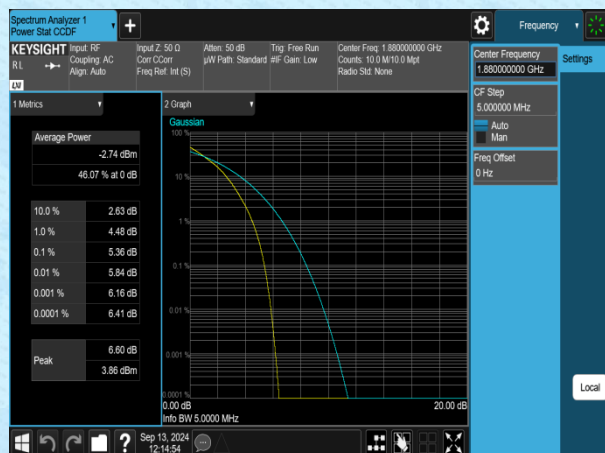
Band2-5MHz-QPSK-18900-1RB#0-PASS
