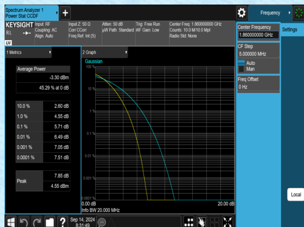
Band2-20MHz-QPSK-18700-1RB#0-PASS
