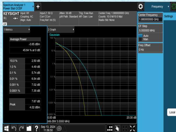
Band2-3MHz-QPSK-18900-15RB#0-PASS
