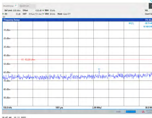
Band41-20MHz-QPSK-39750-1RB#0-Range2:0.15~30MHz
