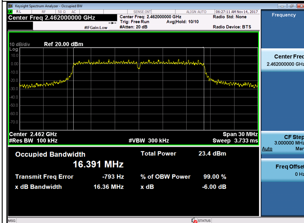
802.11g-2462MHz
