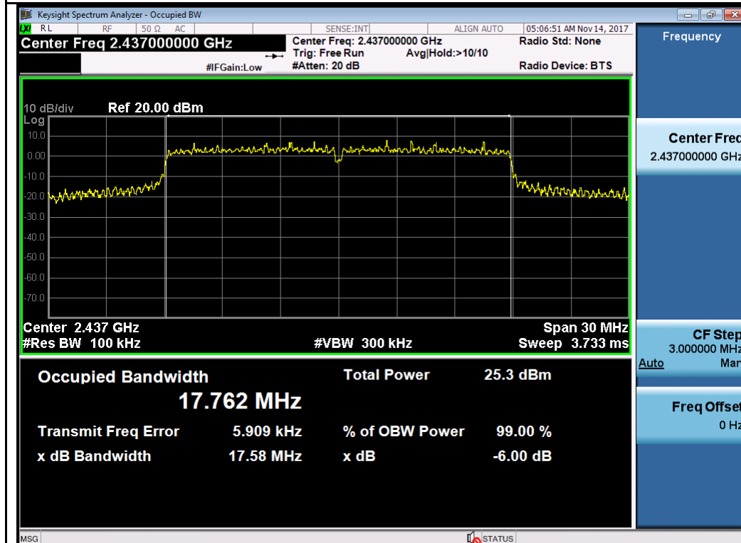
802.11n-HT20-2437MHz
