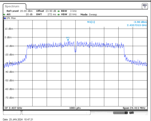
MIMO Ant 6
