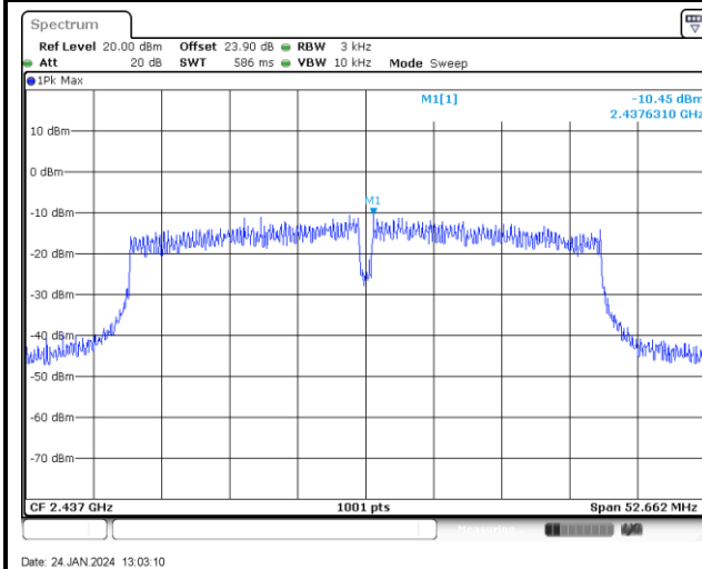
MIMO Ant 3
