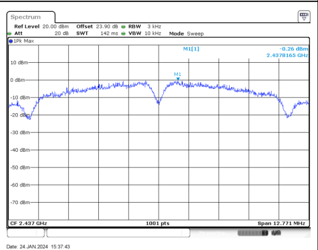
MIMO Ant 6
