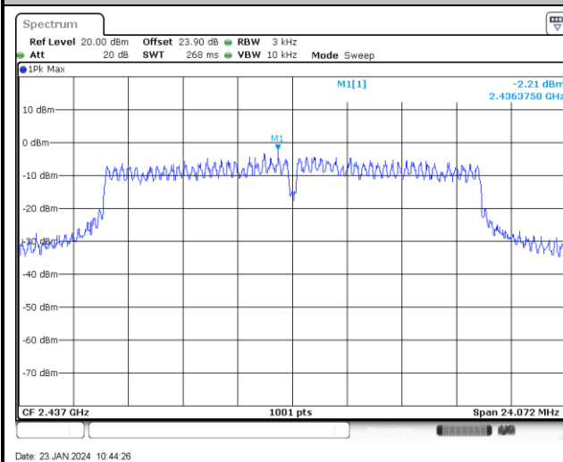
MIMO Ant 3
