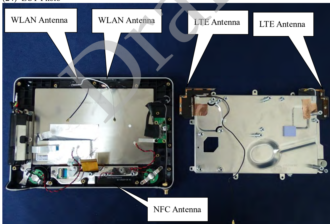
(24) EUT Photo
