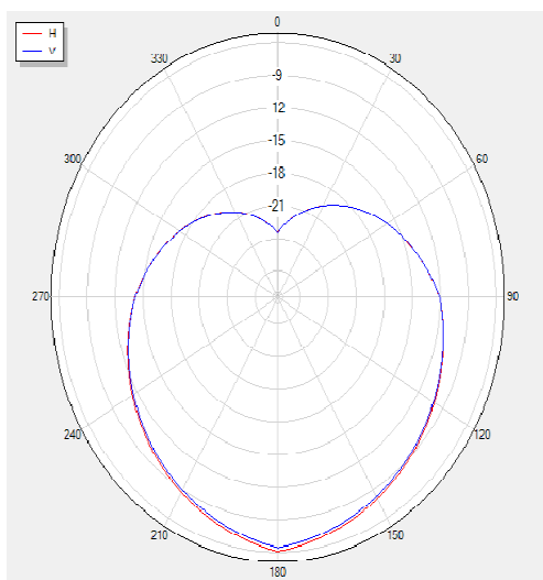
2450 Polar
