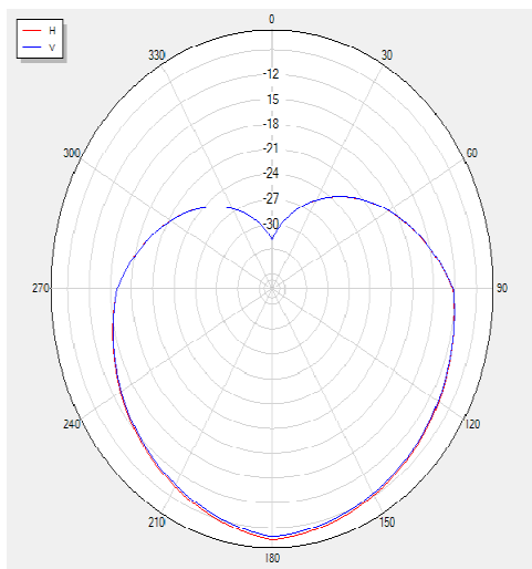
2425 Polar
