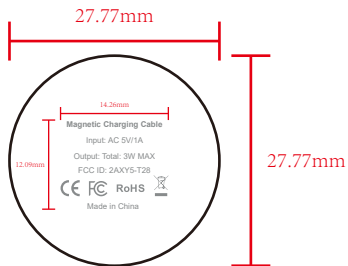
背面丝印
