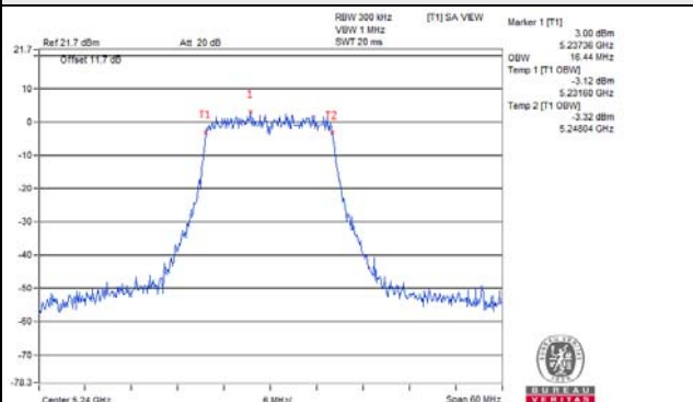
802.11ax (HE20) / Chain 1 / CH 48
