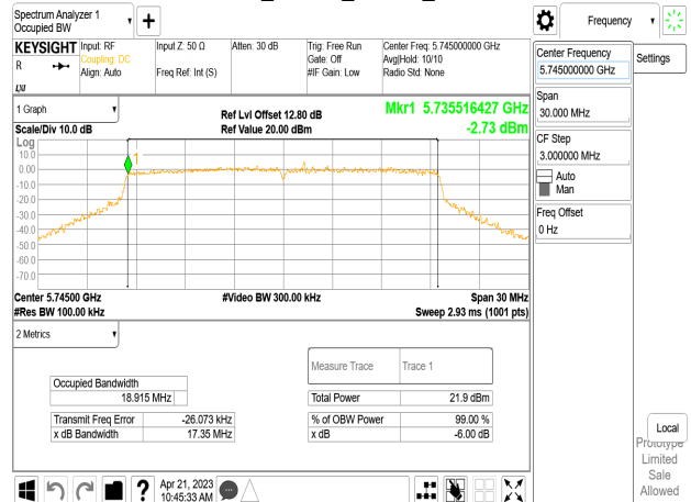
802.11ax_20MHz_Chain1_5745MHz
