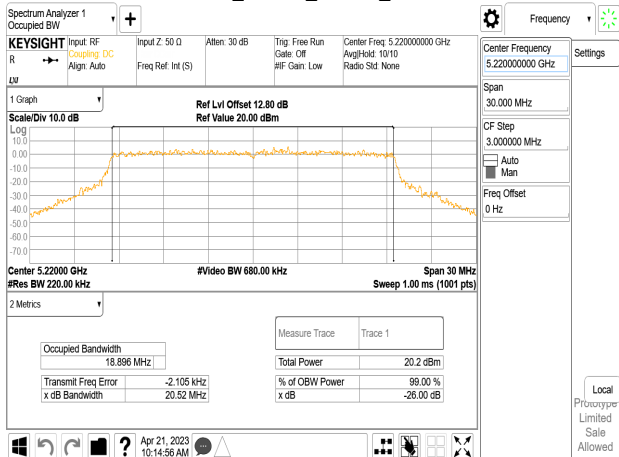
802.11ax_20MHz_Chain1_5220MHz
