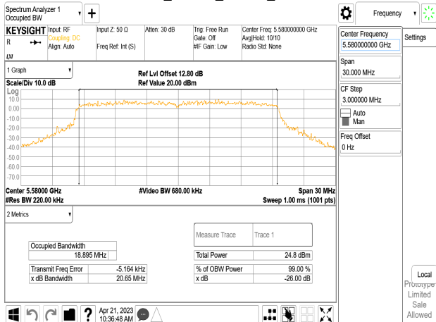
802.11ax_20MHz_Chain1_5580MHz
