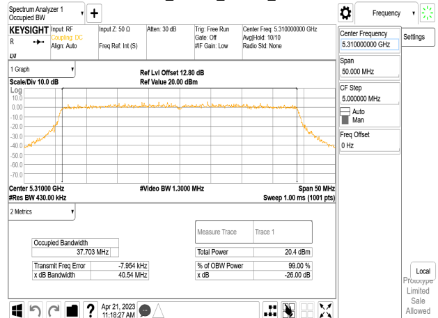
802.11ax_40MHz_Chain0_5310MHz
