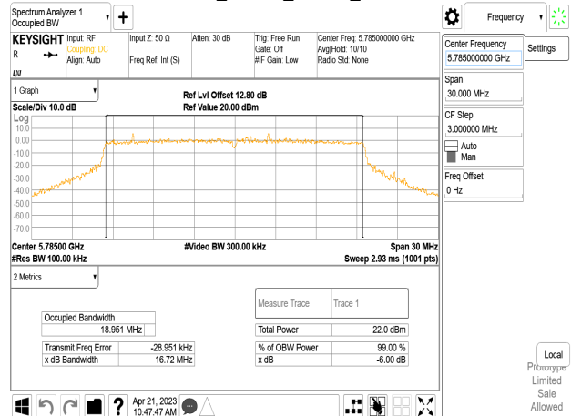
802.11ax_20MHz_Chain0_5785MHz
