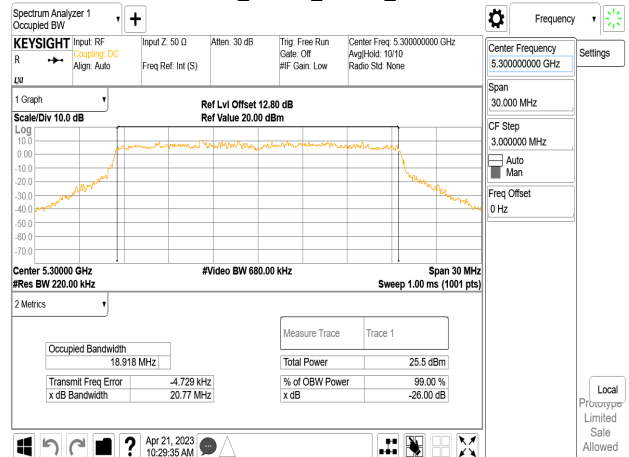
802.11ax_20MHz_Chain1_5300MHz
