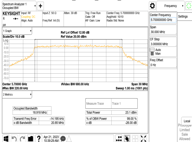
802.11ax_20MHz_Chain0_5700MHz
