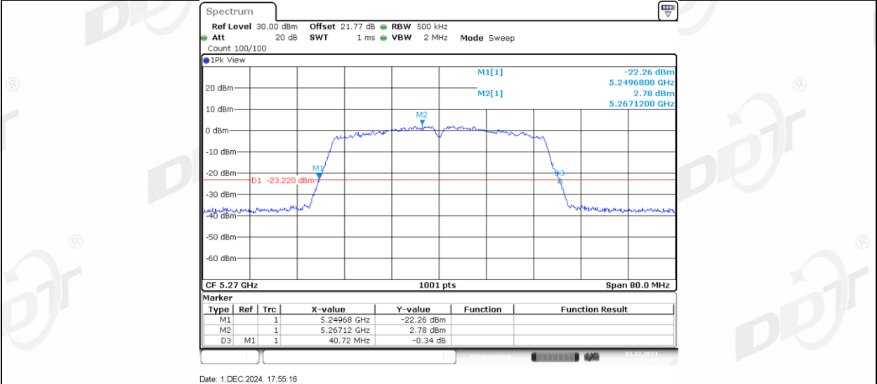
11N40MIMO_Ant2_5270
