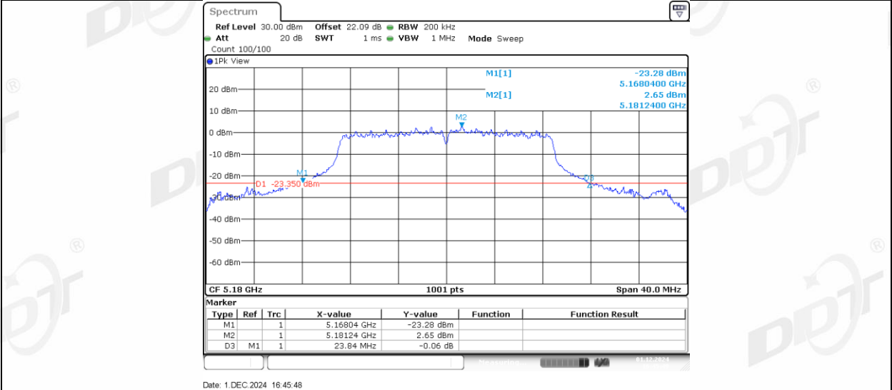
11N20MIMO_Ant2_5180
