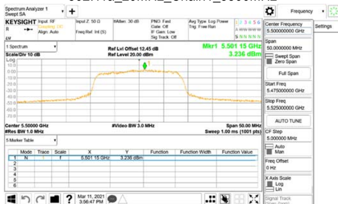
802.11a_20MHz_Chain1_5500MHz
