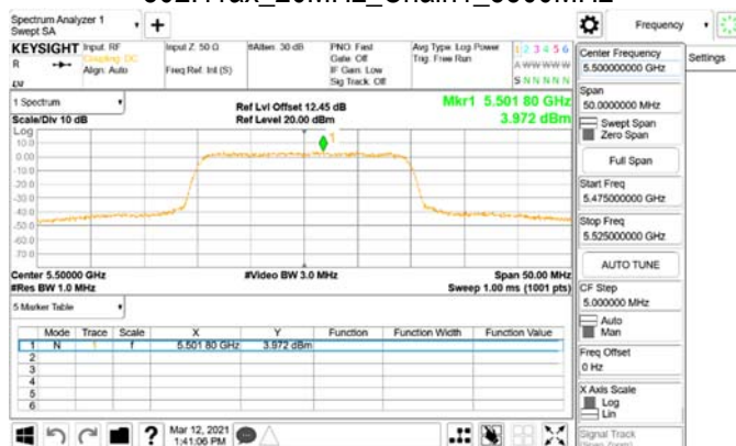
802.11ax_20MHz_Chain1_5500MHz_RU106_53
