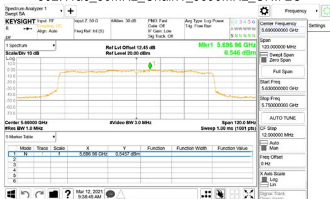
802.11ac_80MHz_Chain1_5690MHz_UNII 2C
