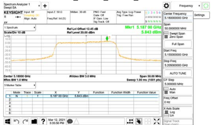
802.11ax_20MHz_Chain1_5180MHz_RU106_53
