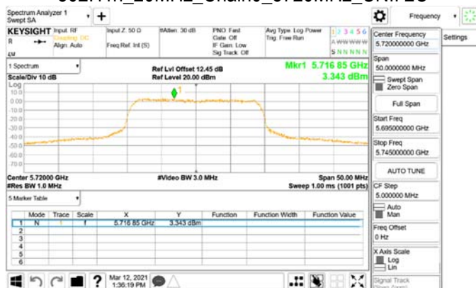
802.11n_20MHz_Chain0_5720MHz_UNII 3
