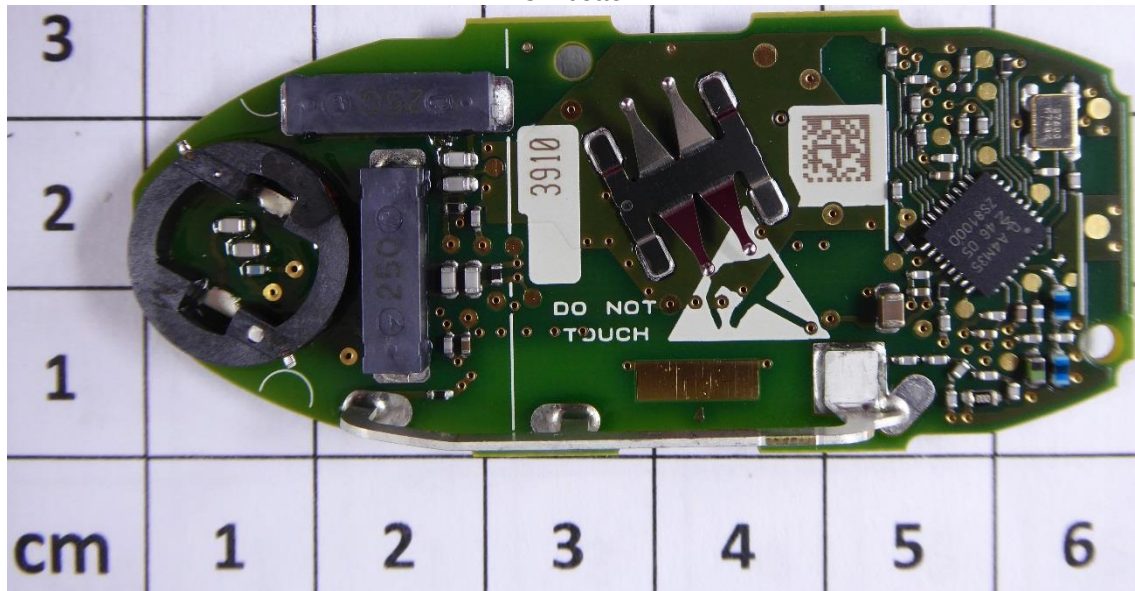
PCB bottom
