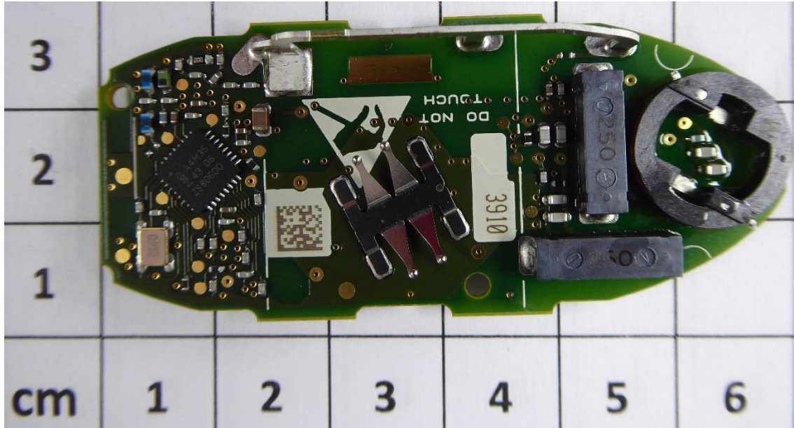
PCB bottom
