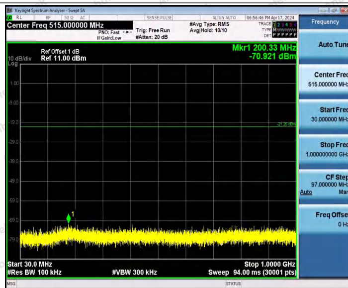
BLE_2M-Ant1-2480-30~1000-PASS
