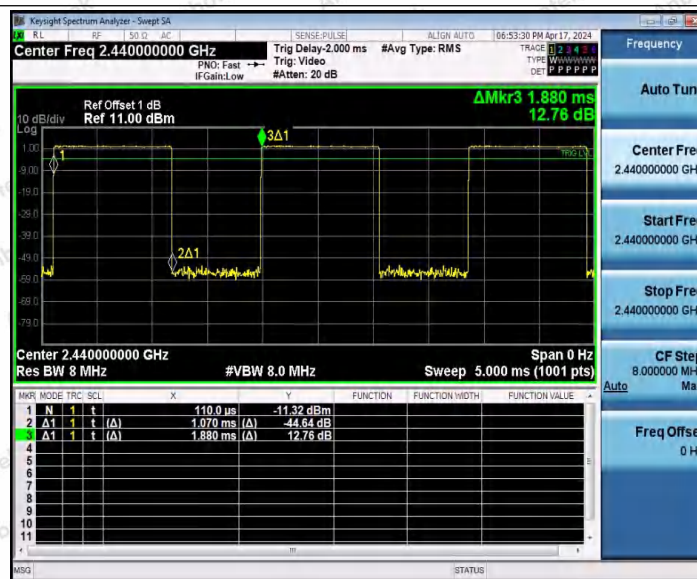
NTNV-BLE_2M-Ant1-2440
