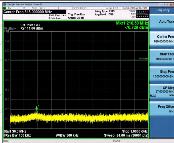
BLE_2M-Ant1-2440-30~1000-PASS
