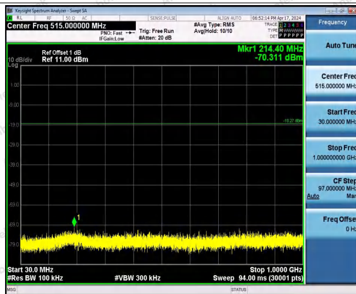
BLE_2M-Ant1-2402-30~1000-PASS
