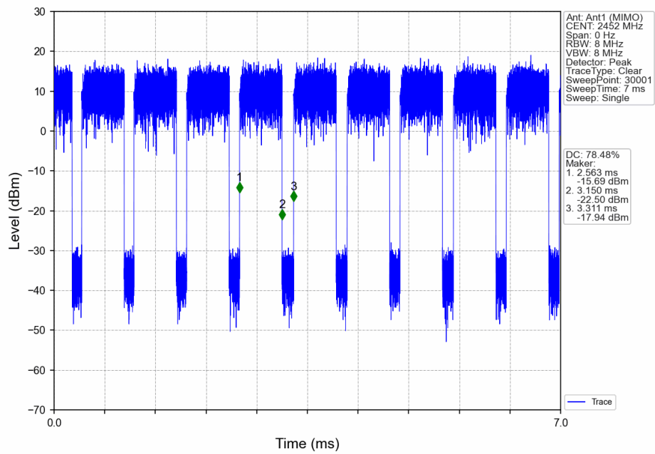
802.11ax(HEW40)_HCH_2452MHz_RU484_Left_Ant1 (MIMO)_NTNV
