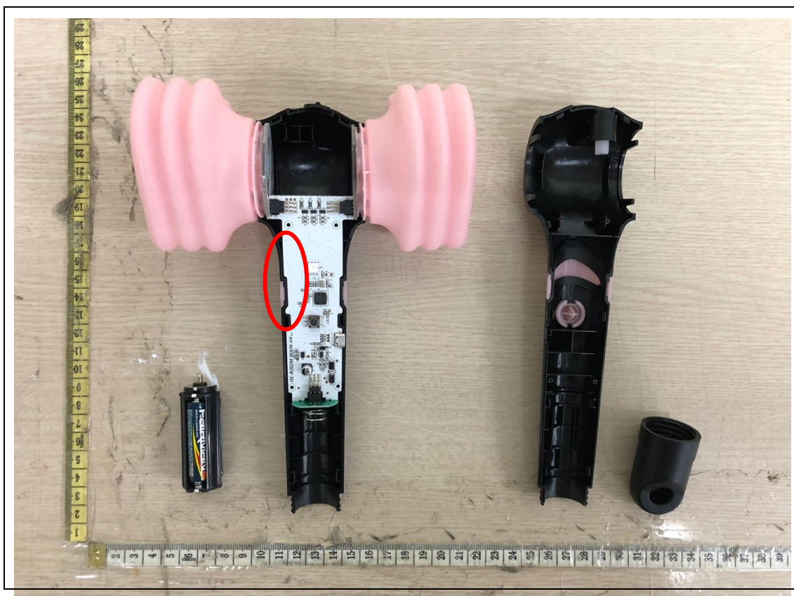
Antenna
