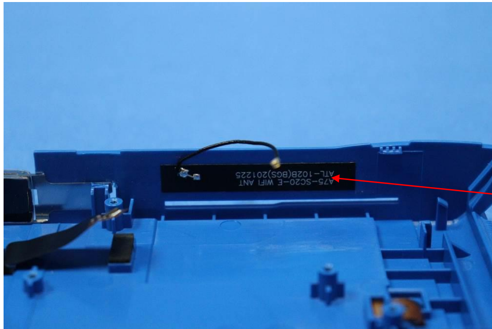
BT/WIFI Antenna
