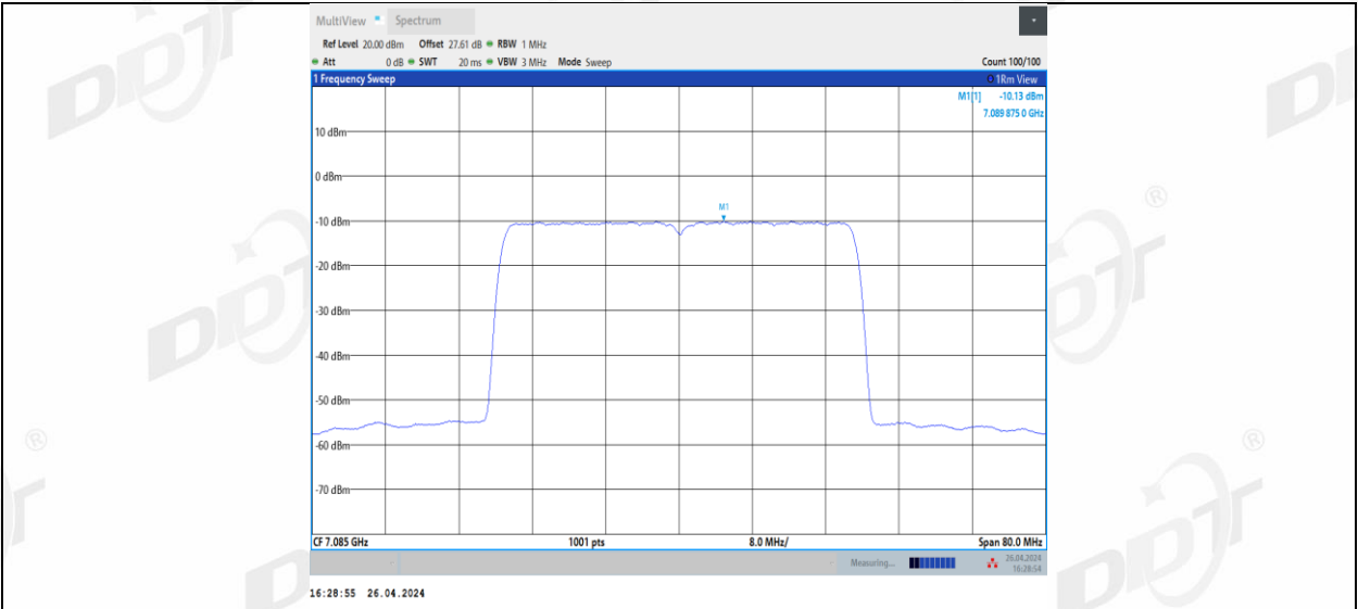
11AX40MIMO_Ant2_7085
