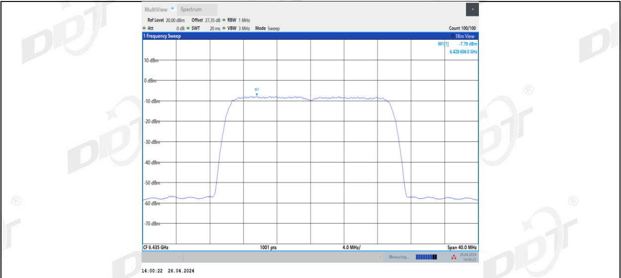
11BE20MIMO_Ant2_6435
