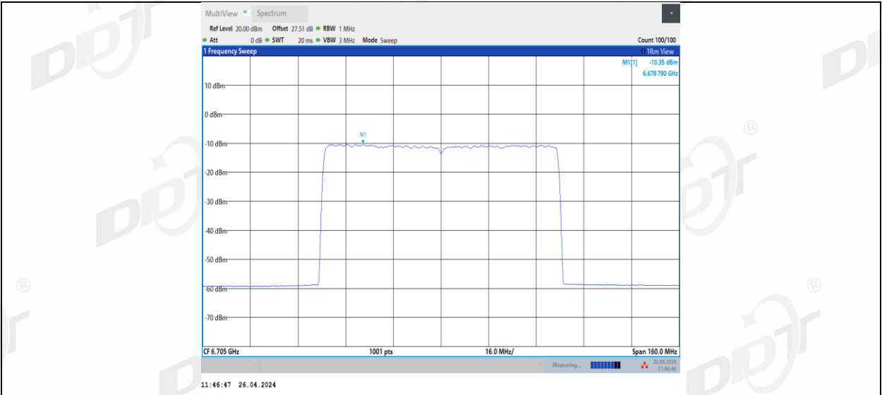
11AX80MIMO_Ant2_6705
