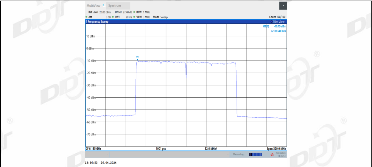
11AX160MIMO_Ant2_6185
