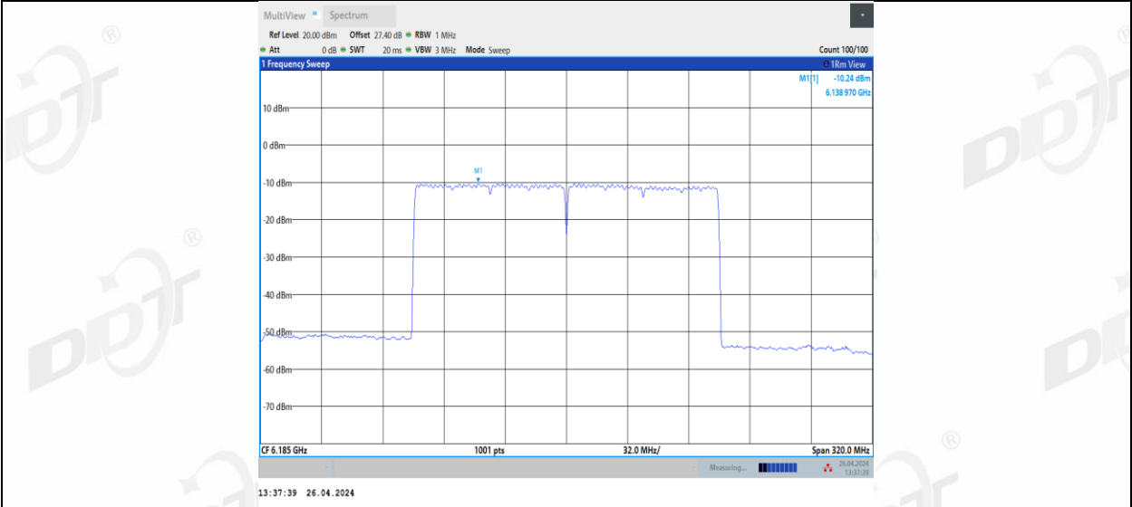
11AX160MIMO_Ant3_6185
