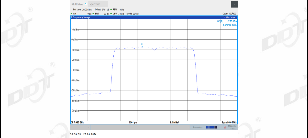
11AX40MIMO_Ant3_7085
