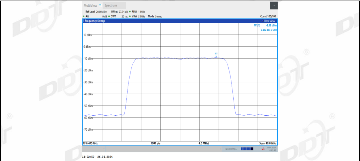
11BE20MIMO_Ant2_6475
