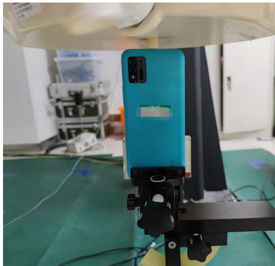
Top(10mm)
