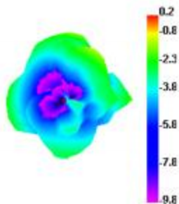
2400.000MHz
