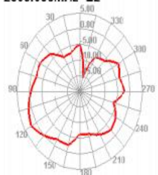
2500.000MHz E2
