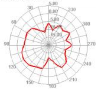
2400.000MHz E2
