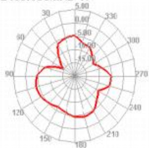
2400.000MHz H
