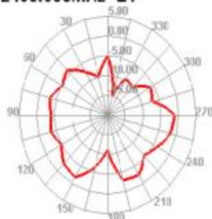
2450.000MHz E1
