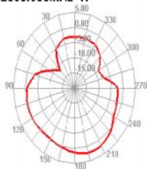
2500.000MHz H
