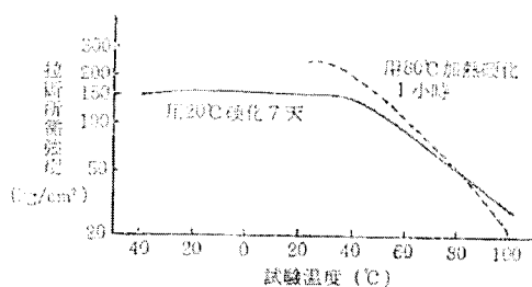
圖II 2.5 耐熱特性 硬化劑混合率爲 100phr
