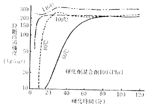
圖II 2.4 加熱硬化特性 硬化劑混合率爲 100phr
