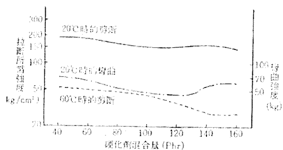
圖II 2.1 硬化劑混合量と粘り強度 (在20°C七天的硬化) 試驗片：軟質板 (25×100×1.6mm) (Over-lap)12.5mm
