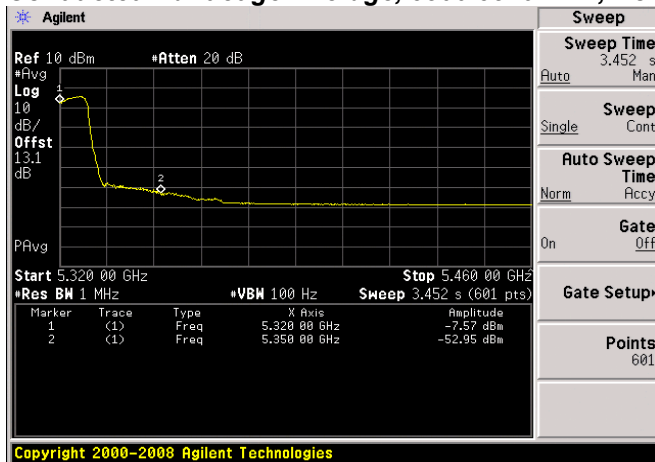
Antenna A
