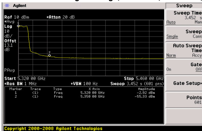
Antenna A
