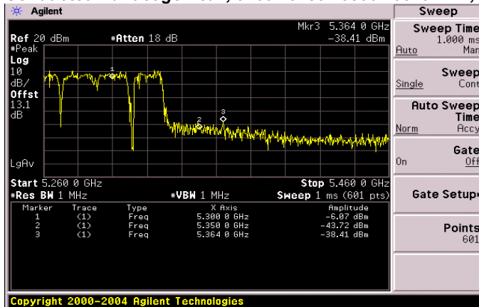
Antenna A
