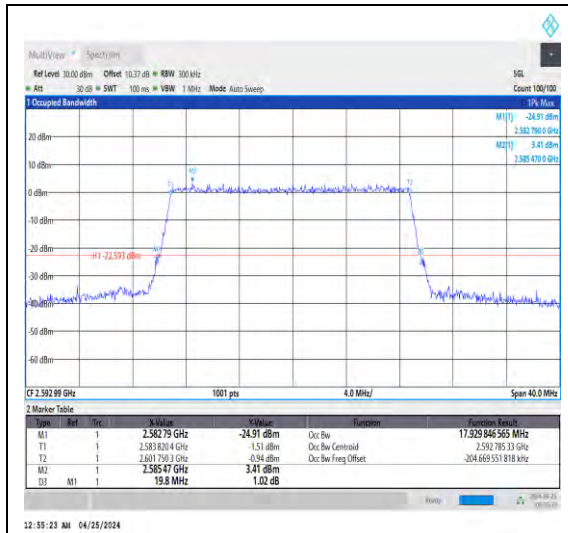
1-N41-30-20-M-5-DFT-256QAM-Out_ Full-50@0-Ant1-17.93-19.800-≤20-PASS
