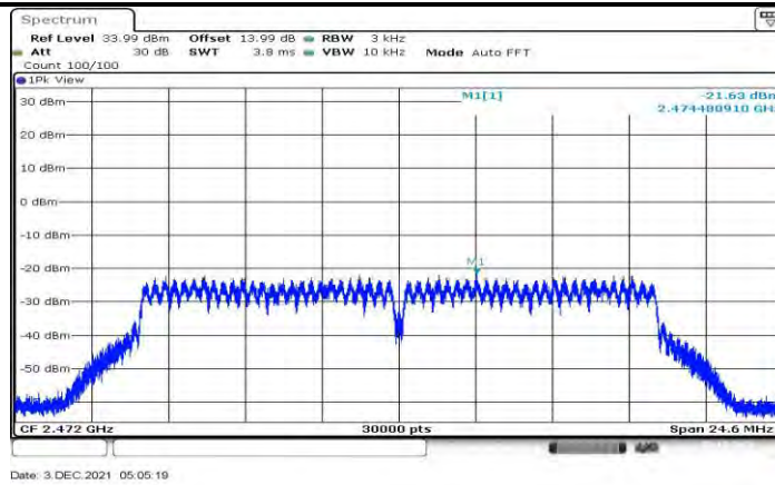
11G Ant1 2472
