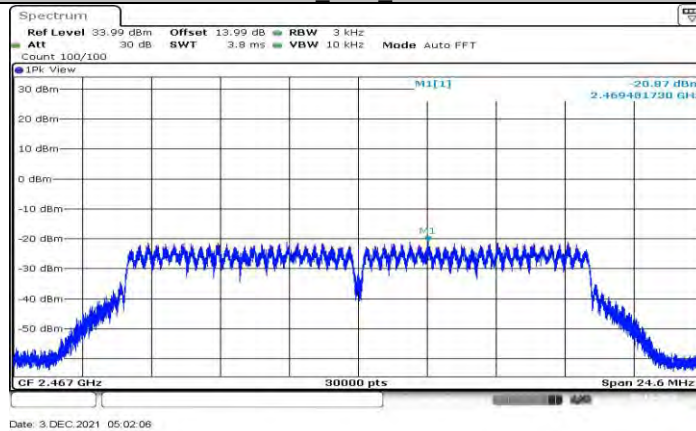
11G_Ant1_2467
