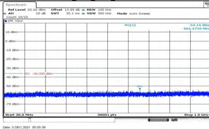
11G_Ant1_2472_30~1000
