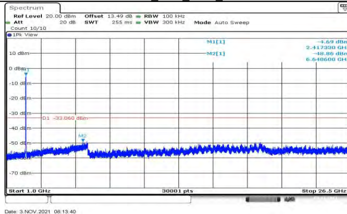
11N20SISO Ant1 2412 1000~26500
