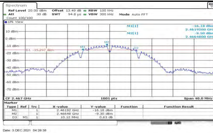
11B Ant1 2467
