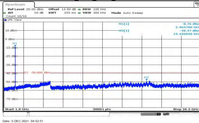
11B_Ant1_2467_1000~26500
