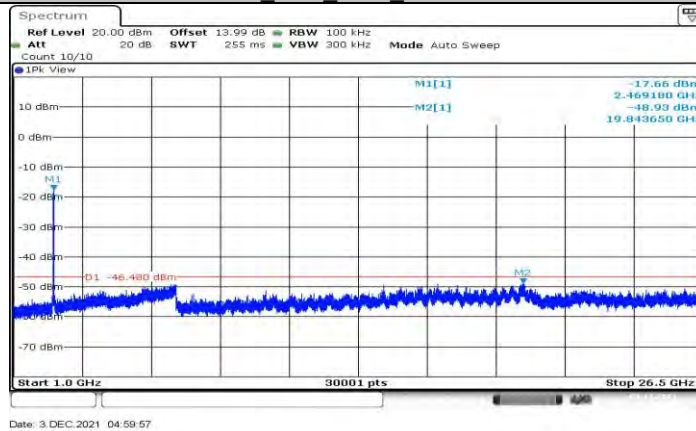
11B_Ant1_2472_1000~26500
