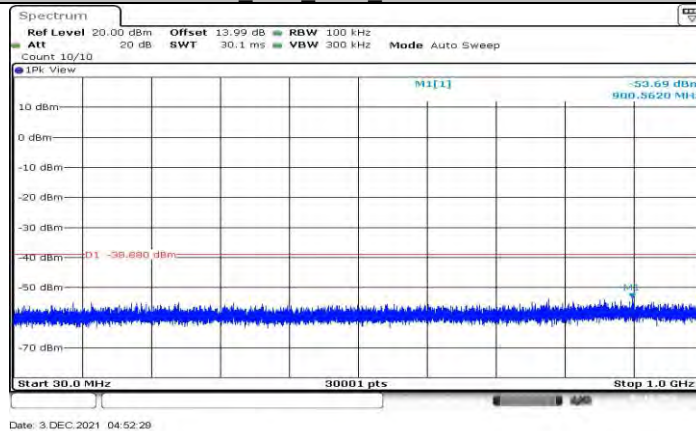
11B_Ant1_2467_30~1000
