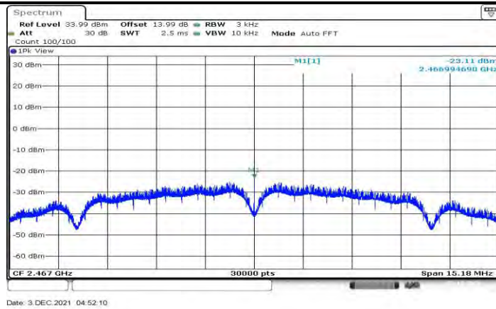
11B Ant1 2467
