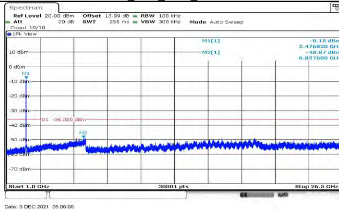
11G_Ant1_2472_1000~26500
