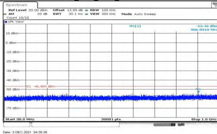
11B_Ant1_2472_30~1000
