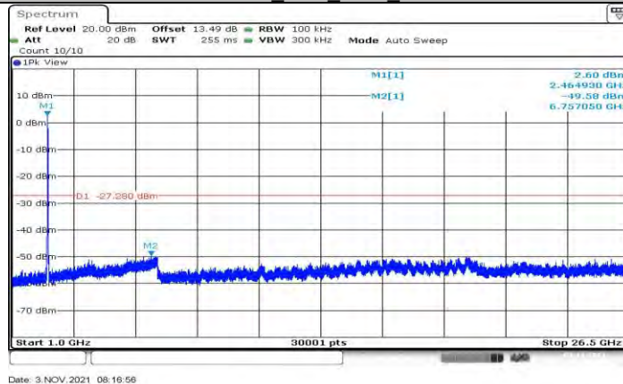
11N20SISO Ant1 2462 1000~26500
