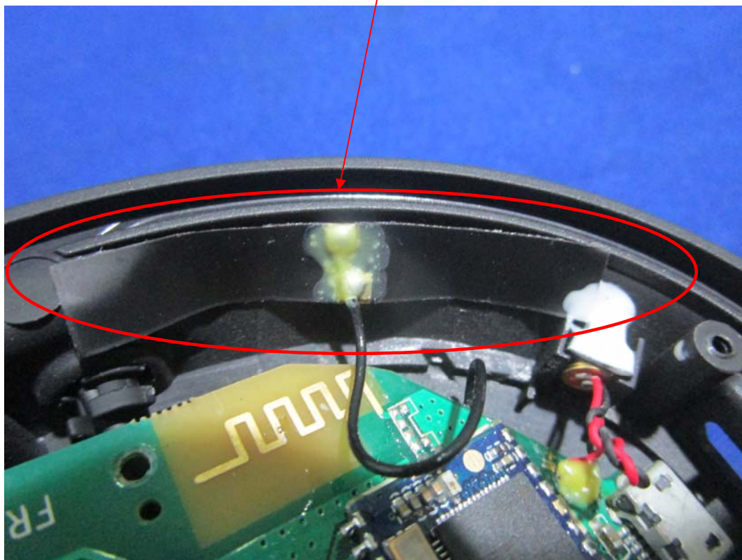
Antenna(FPC)
