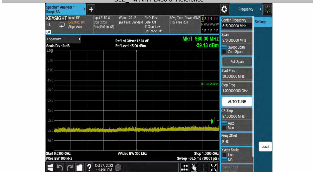
BLE 1M-Ant1-2480-30~1000
