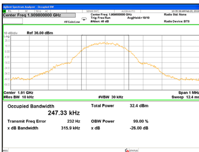
PCS 1900 CH 810
