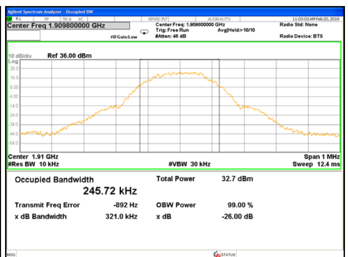
GPRS 1900 CH 810
