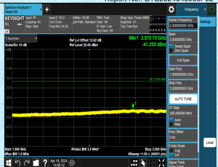
Band5 5MHz QPSK 20625 1RB#0 1000~3000 1000~3000
