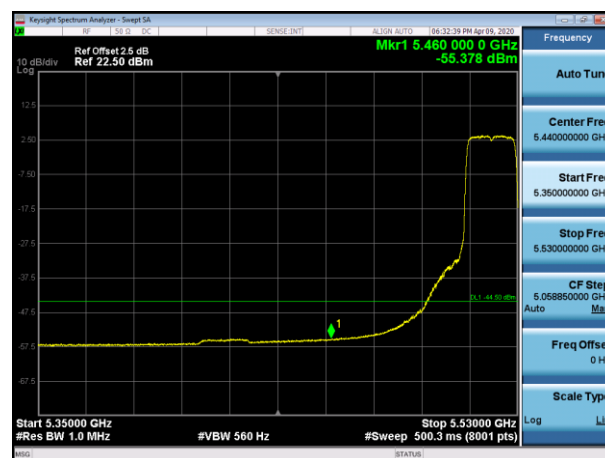
5520MHz AV
