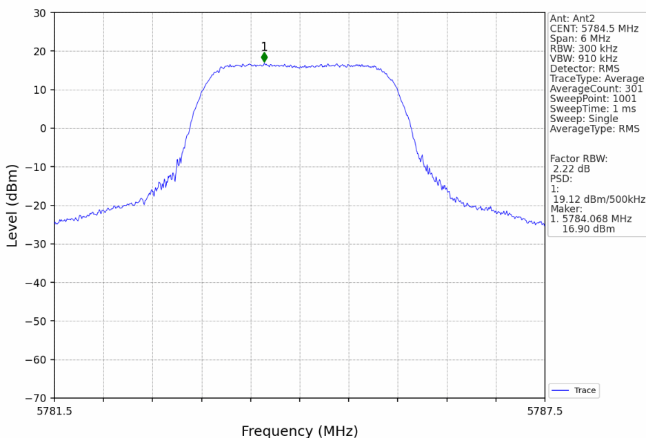
3M_MCH_5784.5MHz_Ant2_NTNV
