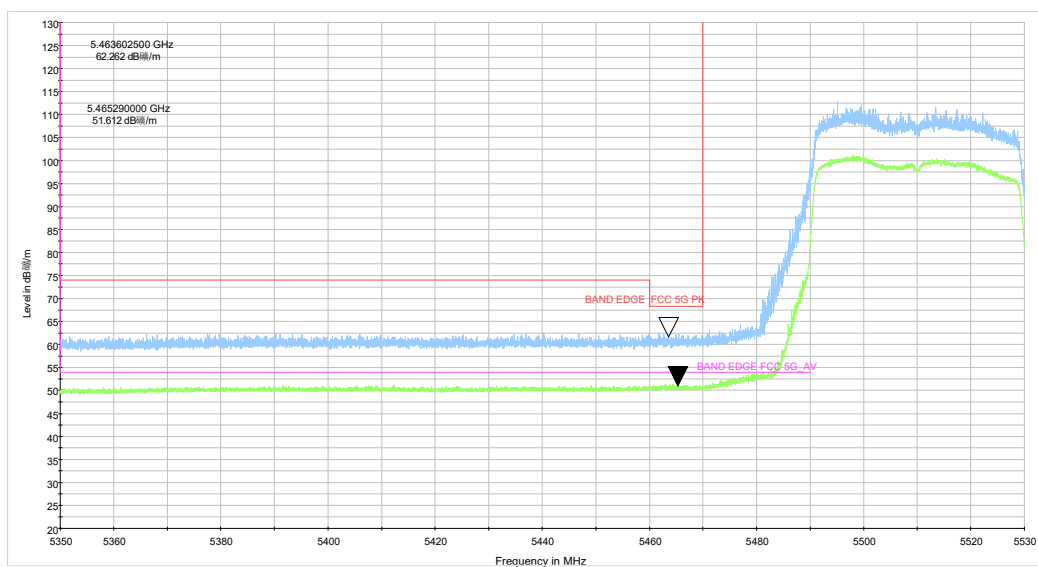
be40 CH102_5.35-5.53GHz_TP14
