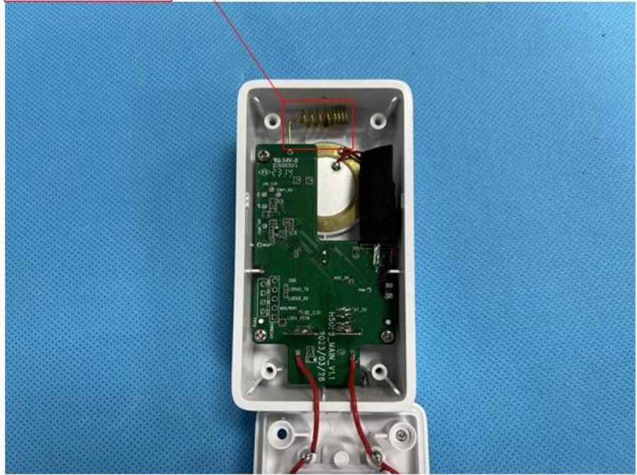
900MHz Antenna
