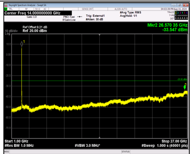
41-41-20MHz-5MHz-QPSK-QPSK-39750-39867-100RB#0-25RB#0-1000~27000MHz-PASS
