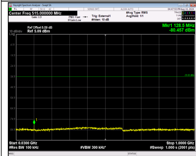
41-41-20MHz-10MHz-QPSK-QPSK-39750-39894-1RB#0 -ORB#0-30~1000MHz-PASS
