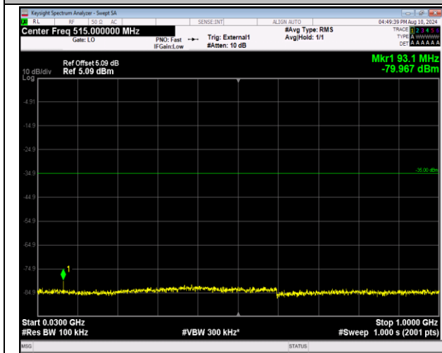
41-41-20MHz-10MHz-QPSK-QPSK-39750-39894-1RB#9 9-0RB#0-30~1000MHz-PASS
