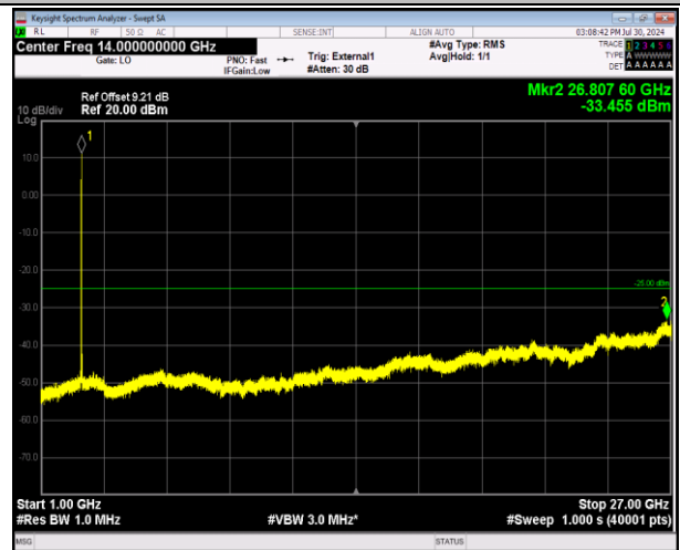
41-41-5MHz-20MHz-64QAM-64QAM-41373-41490-1RB#0- 1RB#99-1000~27000MHz-PASS
