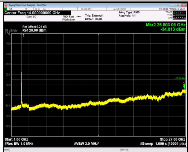
41-41-20MHz-10MHz-QPSK-QPSK-39750-39894-1RB#0-0 RB#0-1000~27000MHz-PASS
