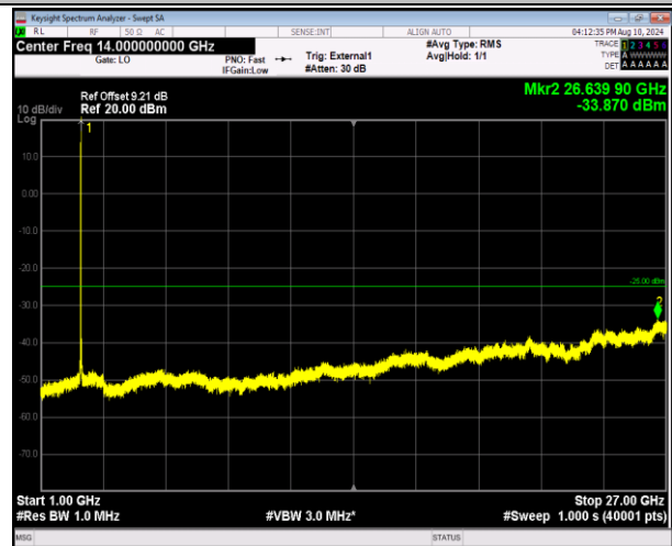
41-41-20MHz-5MHz-QPSK-QPSK-41440-41557-1RB#0-ORB#0-1000~27000MHz-PASS
