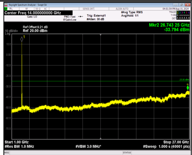
41-41-20MHz-5MHz-QPSK-QPSK-39750-39867-1RB#0-1RB#24-1000~27000MHz-PASS
