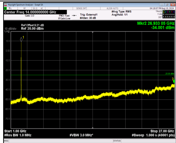
41-41-20MHz-5MHz-QPSK-QPSK-41440-41557-100RB#0-25RB#0-1000~27000MHz-PASS
