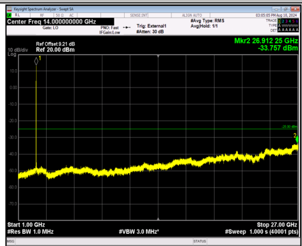
41-41-5MHz-20MHz-16QAM-16QAM-41373-41490-1RB#0- 1RB#99-1000~27000MHz-PASS
