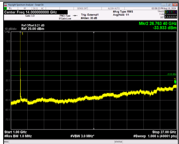
41-41-20MHz-5MHz-QPSK-QPSK-39750-39867-1RB#0-ORB#0-1000~27000MHz-PASS
