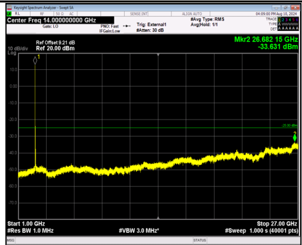
41-41-20MHz-5MHz-QPSK-QPSK-40595-40712-1RB#0-1RB#24-1000~27000MHz-PASS
