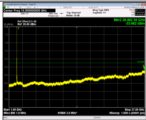
41-41-20MHz-10MHz-QPSK-QPSK-39750-39894-1RB#99- 0RB#0-1000~27000MHz-PASS
