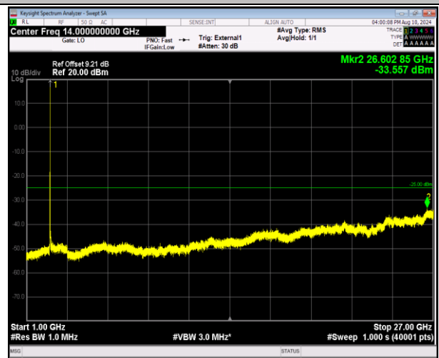
41-41-20MHz-5MHz-QPSK-QPSK-39750-39867-1RB#99-0RB#0-1000~27000MHz-PASS
