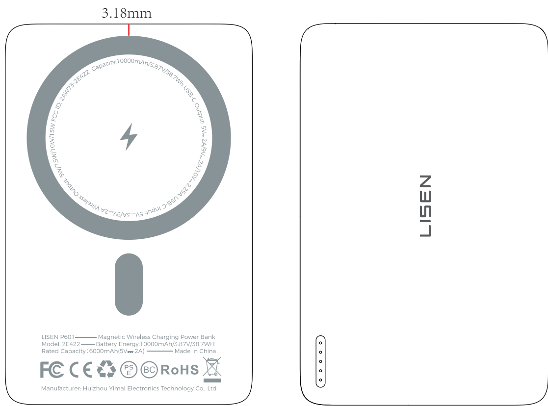
丝印位置分布图示意
