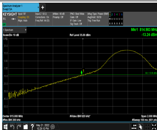
Band18-10MHz-QPSK-23900-1RB#0
