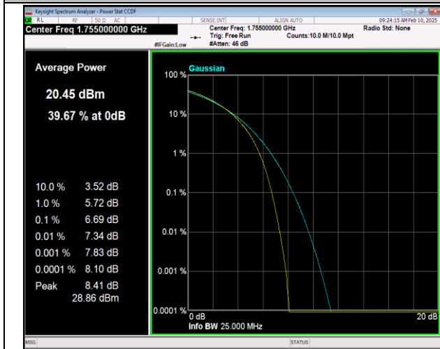
66-66-20MHz-20MHz-QPSK-QPSK-132323-132521-100R B#0-100RB#0-PASS
