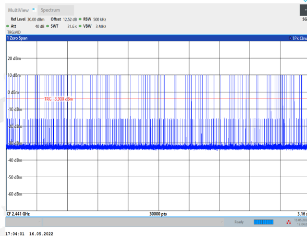
DH5_Ant1_Hop
