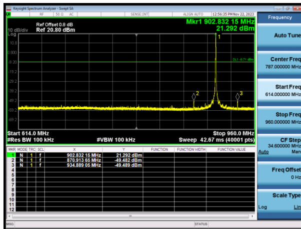
Channel64 903MHz
